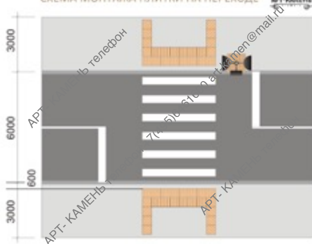
СХЕМА МОНТАЖА ПЛИТКИ НА ПЕРЕХОДЕ
